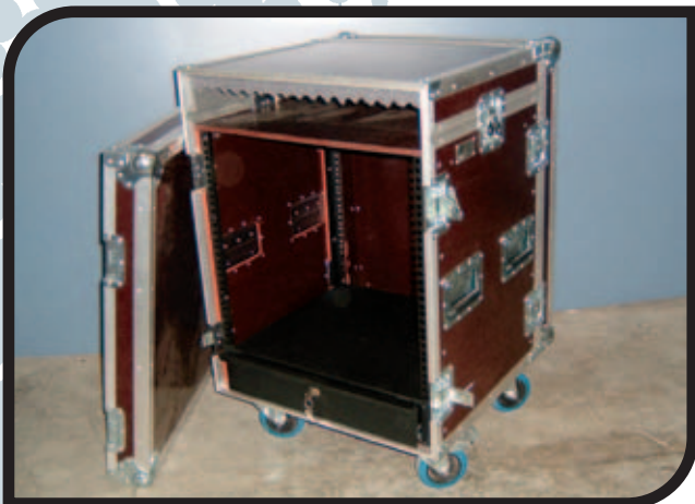
Rack de tres tapas. [Para colocación de mesa].
